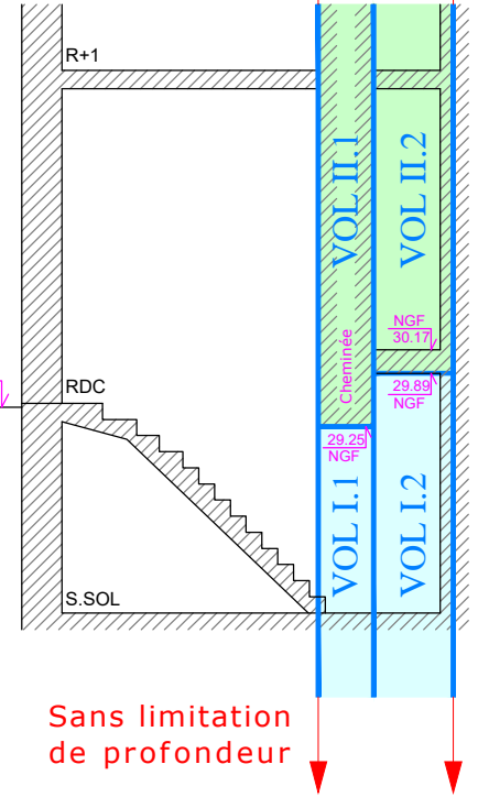
COUPE
